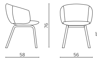
NT 4094 MINI 4 legs wooden base base a 4 gambe in legno
